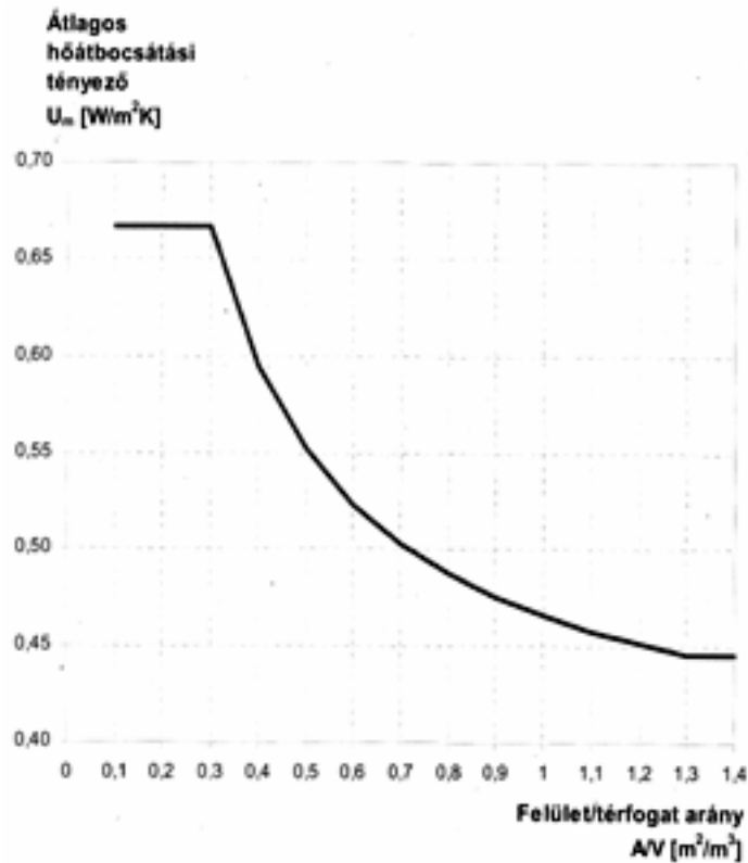
2. ábra: Az átlagos hőátbocsátási tényező követelményértékei
