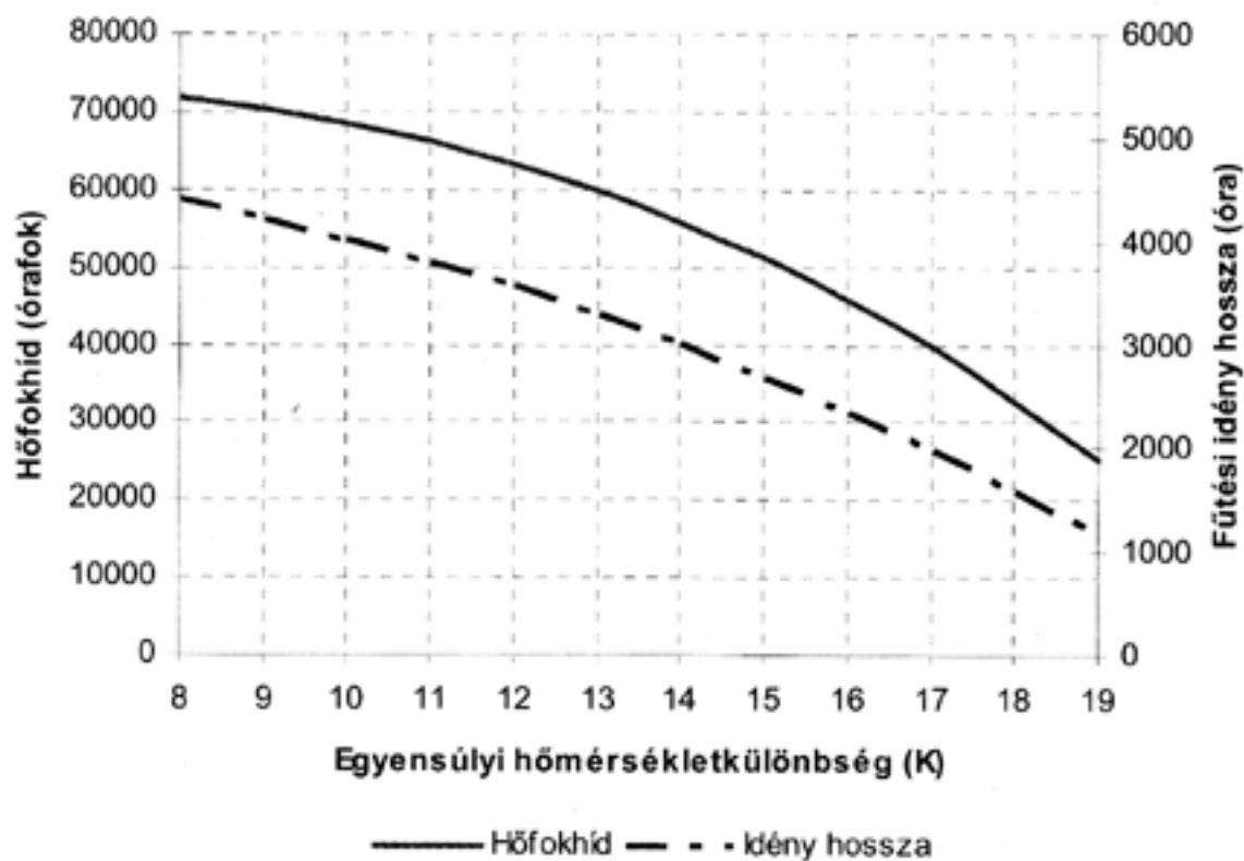
1. ábra: Hőfokhid és fűtési idény hossza 20 °C belső hőmérséklet esetén az egyensúlyi hőmérséklet-különbség függvényében
