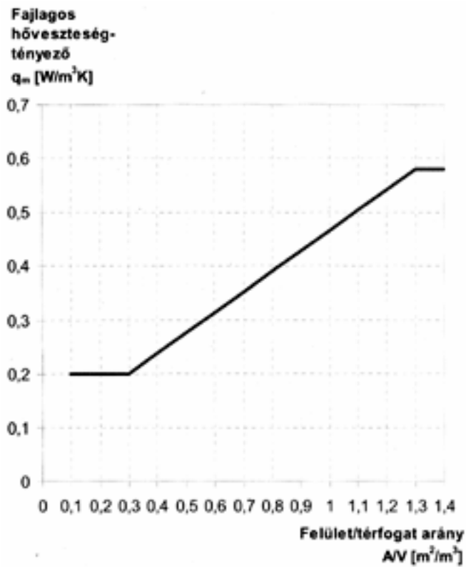
1. ábra: A fajlagos hővesztés-tényező követelményértéke
